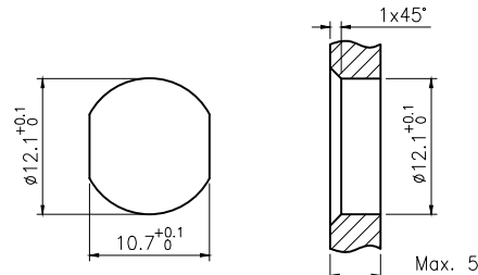
面板开孔尺寸
